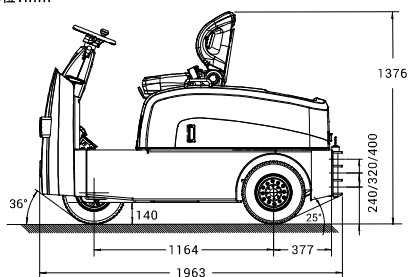
产品外形参数 Vehicle Dimensions
